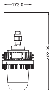
吊掛 90° (H90)
