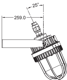
壁掛 25° (W25G)
